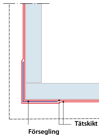
FIGUR 7. Hörn i skivvägg.
